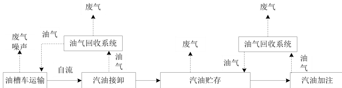
图 2-2 汽油加油工艺流程及产污节点图
